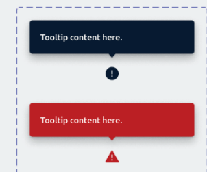
Tooltip
