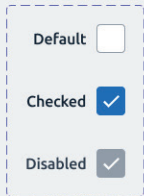
Checkbox
